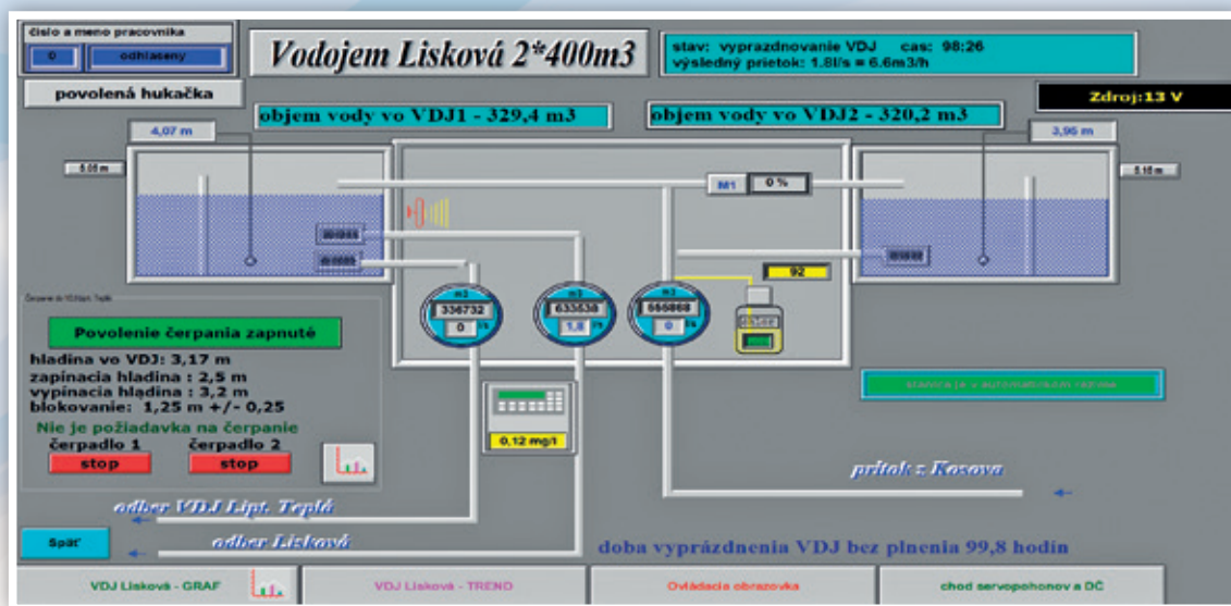
Dispečingový systém – Bloková schéma VDJ Lisková (2x400 m 3 )
