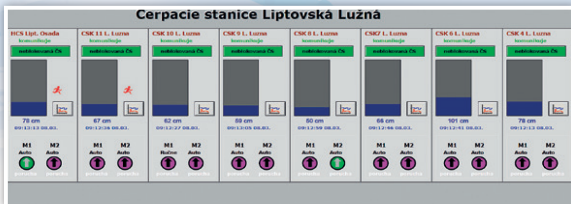
Dispečingový systém – Prehľad čerpacích staníc pri ČOV Liptovská Osada
